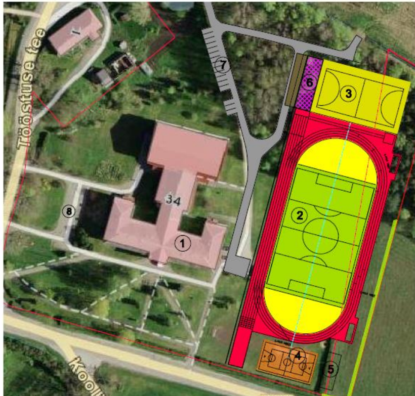
Illustratsioon Võnnu aleviku Tartu tn 34 kinnistu ja lähikümbruse detailplaneeringust
